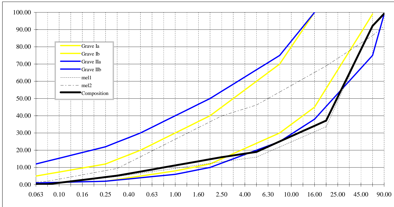
Courbe de composition de la grave selon SN 670 120c
